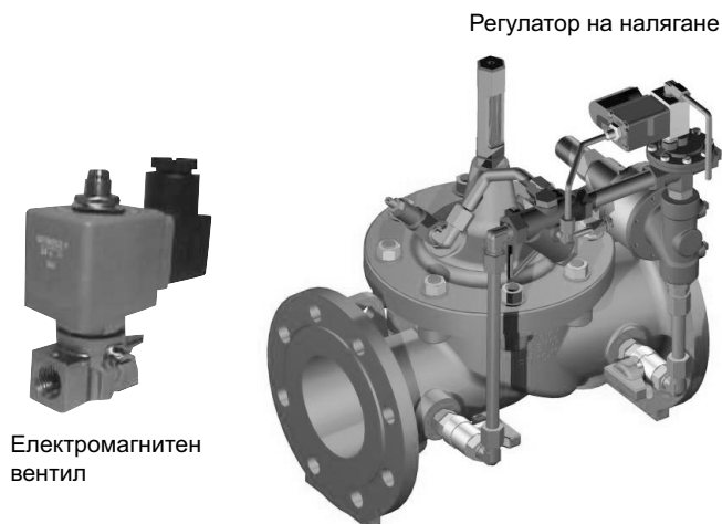
Регулатор на налягане
